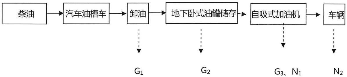
图例：G 废气；N 噪声；S 固废；
