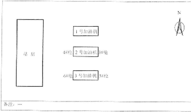
附检测点位示意图
