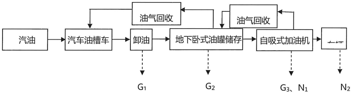
图例：G 废气；N 噪声；S 固废；
